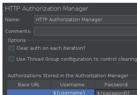
Рисунок 7 – Настройка HTTP Authorization Manager
