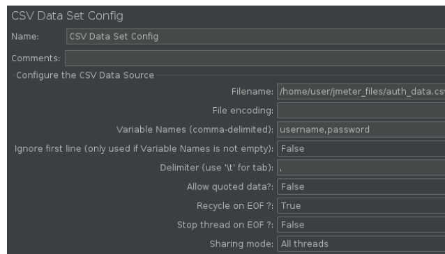
Рисунок 6 – Настройка CSV-источника данных
