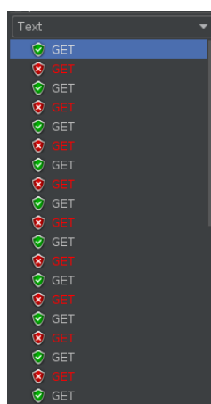
Рисунок 10 – Статусы HTTP-ответов
